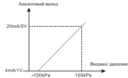
Рис. 4: Аналоговый выход
